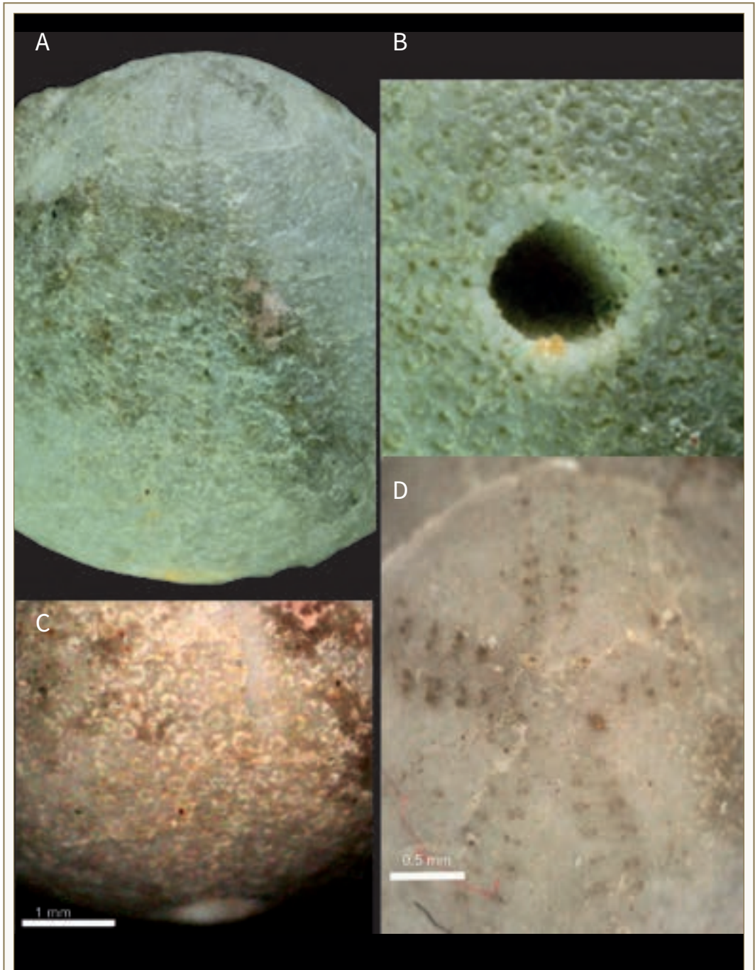
FIGURA 4. Pseudonucleus aff. malladai Lambert, 1920, del Campanià de Loredo (península Ibèrica). MNHN.F.A94628. A: detall ambulacre III, vista anterior. B: detall peristoma i fíl·lodes. C: detall tuberculació zona frontal. D: detall pètals i gonoporus. Fotos A i B de M. Saura.
